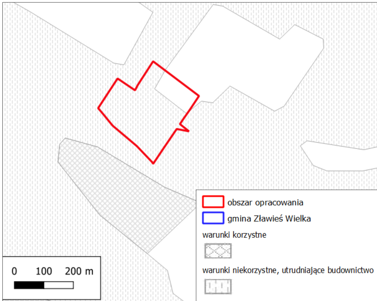
Rysunek 12. Warunki podłoża budowlanego
